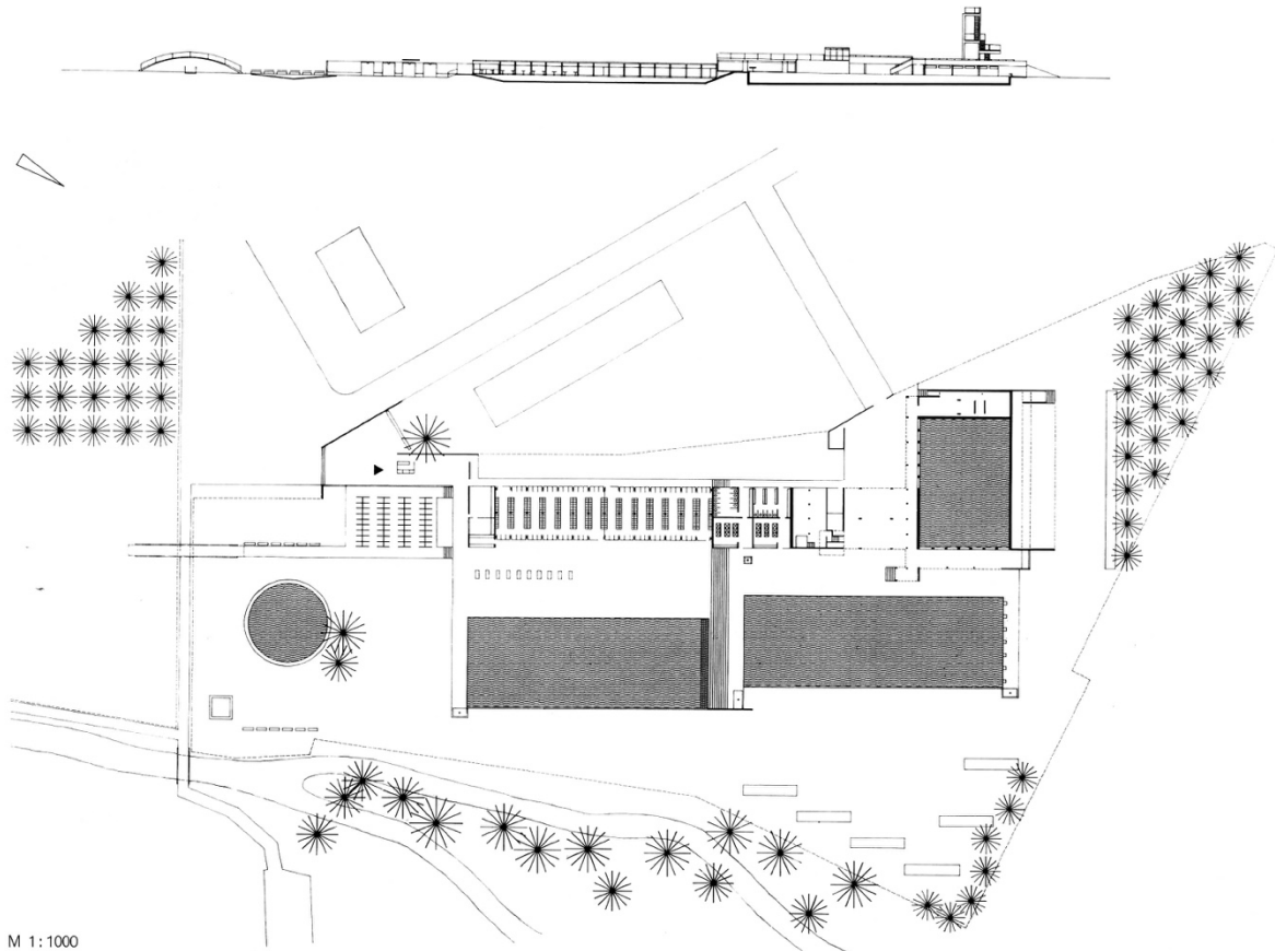
Lageplan Parkbad Ternitz (Roland Rainer Archiv, Az W)
